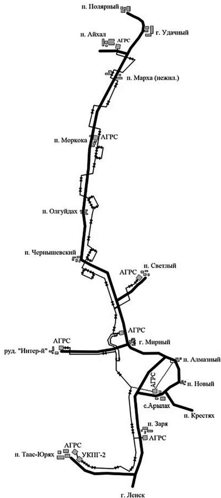
План-схема магистрального газопровода Тас-Юрях – Мирный – Айхал по территории МО «Мирнинский район»
